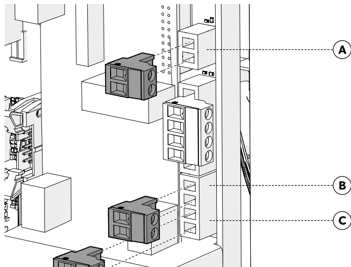
Figuur 33 Het aansluiten van verschillende onderdelen op de besturingsunit (P12).
