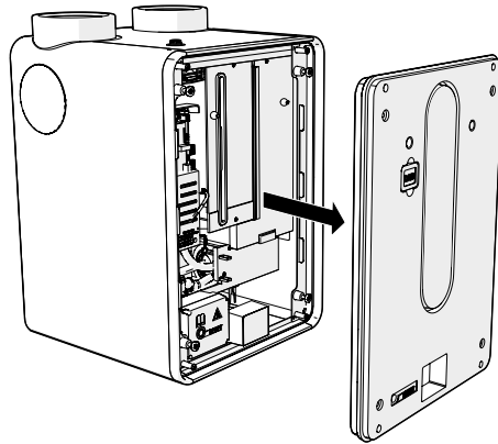
Figuur 43 Het verwijderen van de voorzijde.
