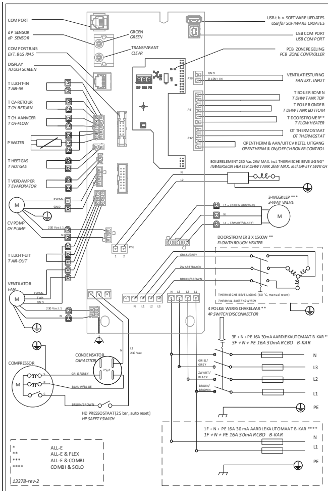
Figuur 31 Elektrisch aansluitschema van de Modul-AIR
