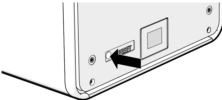
Figuur 49 Het resetten van de doorstromerbeveiliging.
