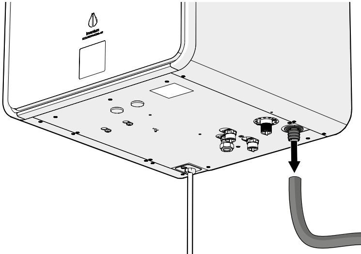
Figuur 45 Het verwijderen van de condensafvoerslang.
