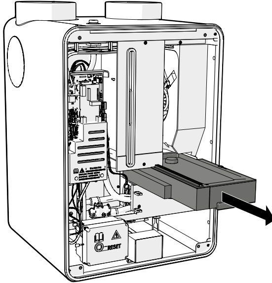
Figuur 47 Het verwijderen van de lekbak uit de Modul-AIR.
