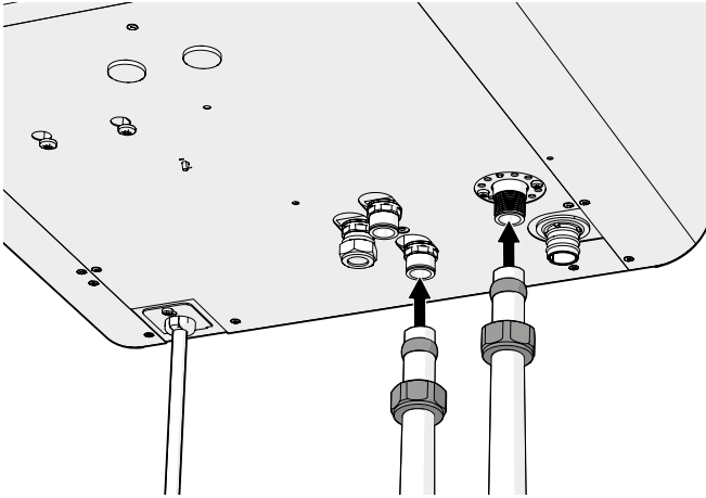
Figuur 25 Het star aansluiten van de cv-leidingen op de Modul-AIR.
