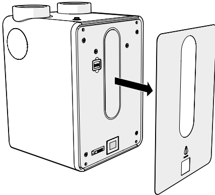
Figuur 41 Het verwijderen van de frontplaat. Figuur 42 De vier los te draaien schroeven.
