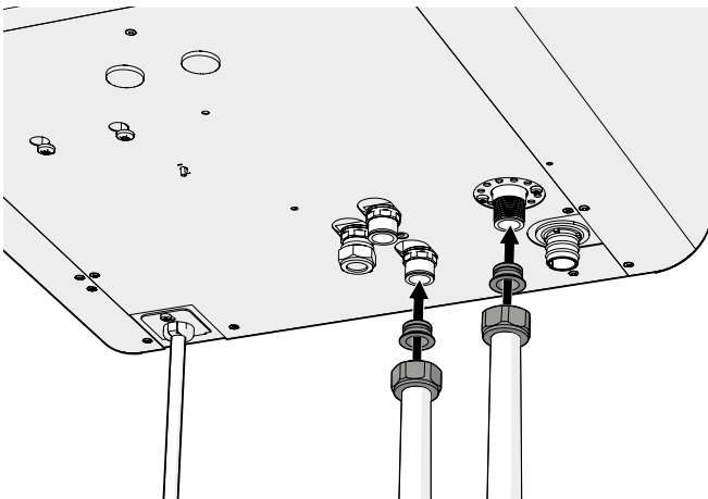
Figuur 26 Het flexibel aansluiten van de cv-leidingen op de Modul-AIR.
