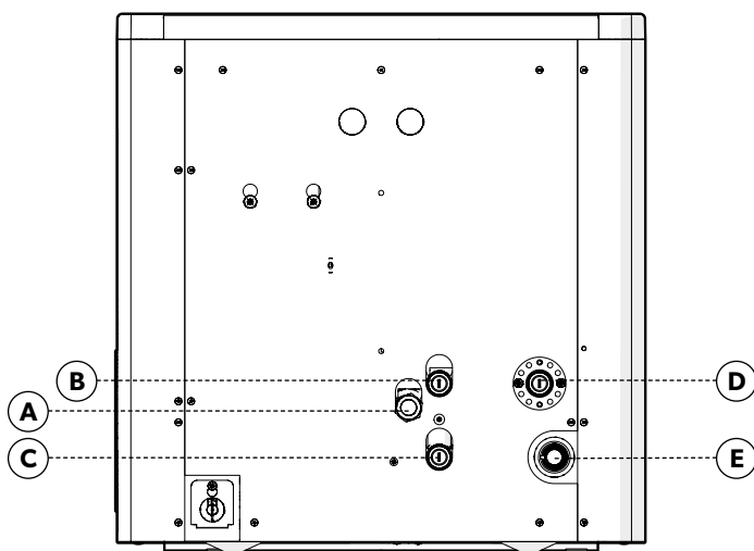
Figuur 22 De aansluitingen op de onderkant van de Modul-AIR.
