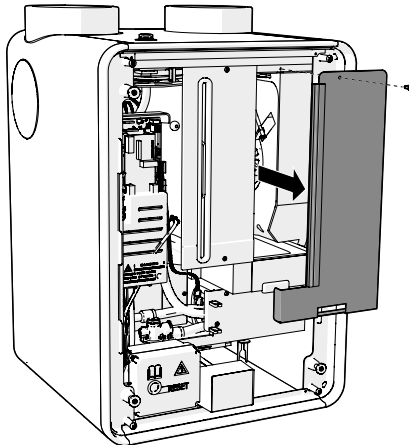
Figuur 44 Het verwijderen van de afdekplaat.
