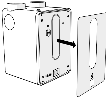
Figuur 48 Het verwijderen van de frontplaat.
