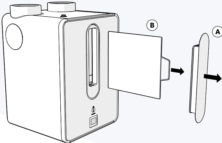
Figuur 40 Het verwijderen van het filter.
