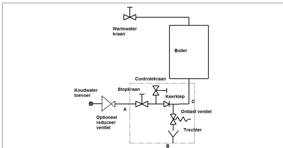
Schema inlaatcombinatie
